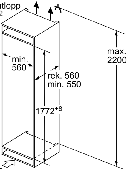
Mått i mm
