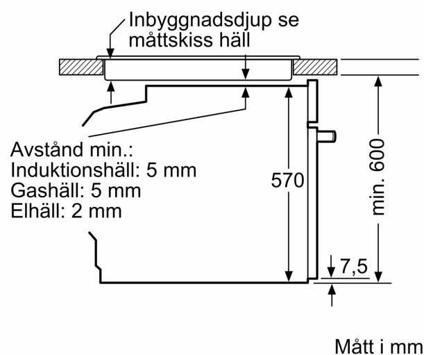
Inbyggnad med håll.
