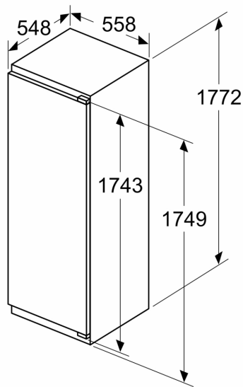
Mått i mm
